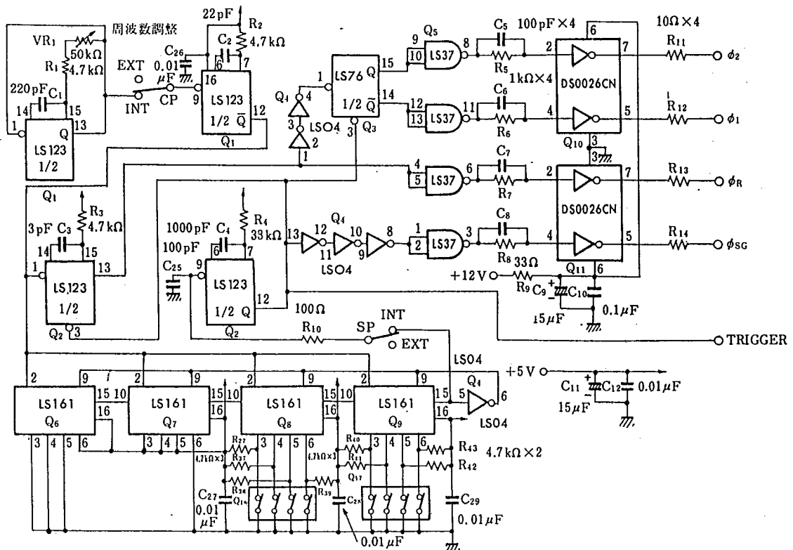
■ 駆動回路図 (デジタル部) / Drive Circuit (Digital)
